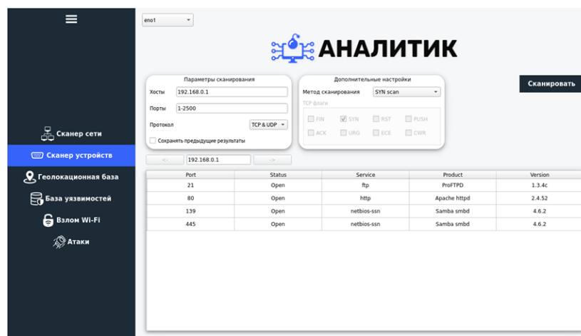
Рис. 2. Результат работы модуля «Сканер устройств»
