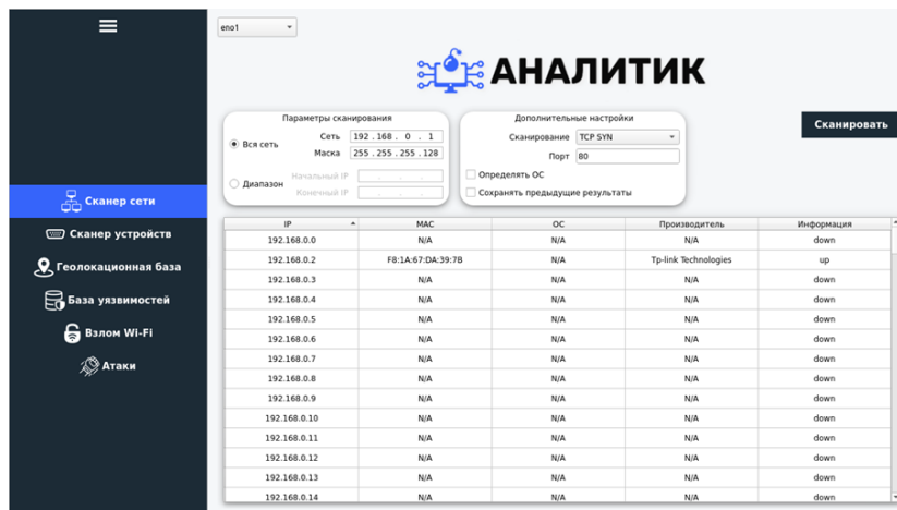
Рис. 1. Результат работы модуля «Сканер сети»
