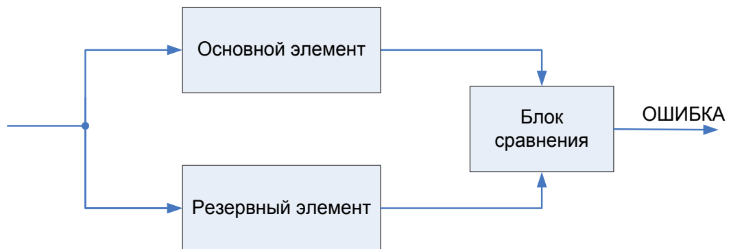
Рисунок. Схема метода дублирования с нагруженным резервным элементом
