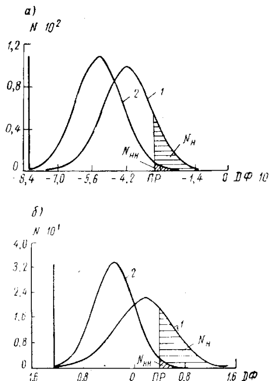
Рис.2 Дискриминационная функция для годных(1) и негодных (2) ИС.
