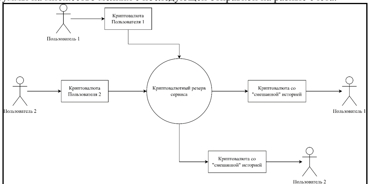
Рис. 1. Схема работы сервисов-«миксеров»
