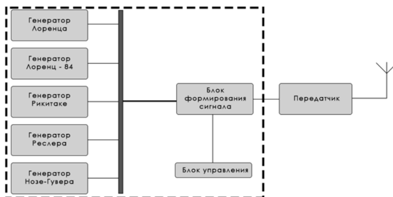
Рис. 2. Структурная схема устройства генератора «Айсберг 2.0»
