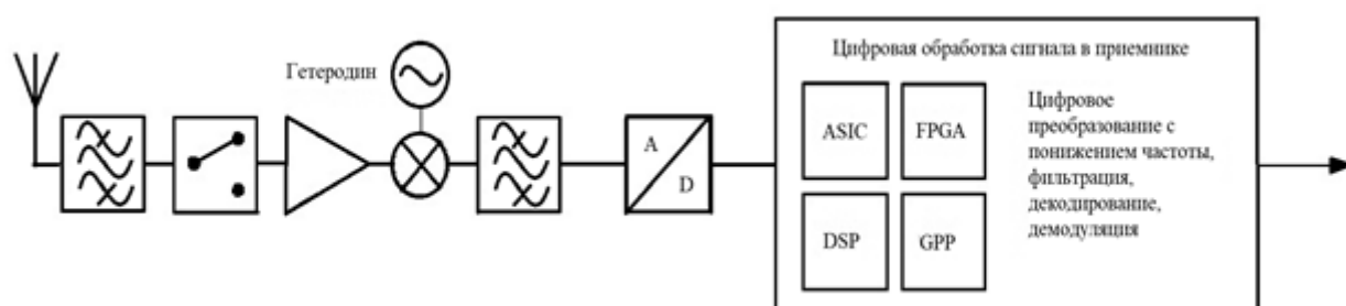
Рис. 1. Функциональная схема программно-определяемого радио
