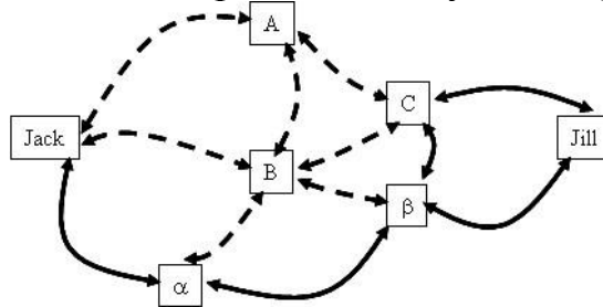
Рис. 1. Маршрутизация MANET через защищенные узлы в момент времени 1 (—) и безопасные узлы в момент времени t_2 (---)
