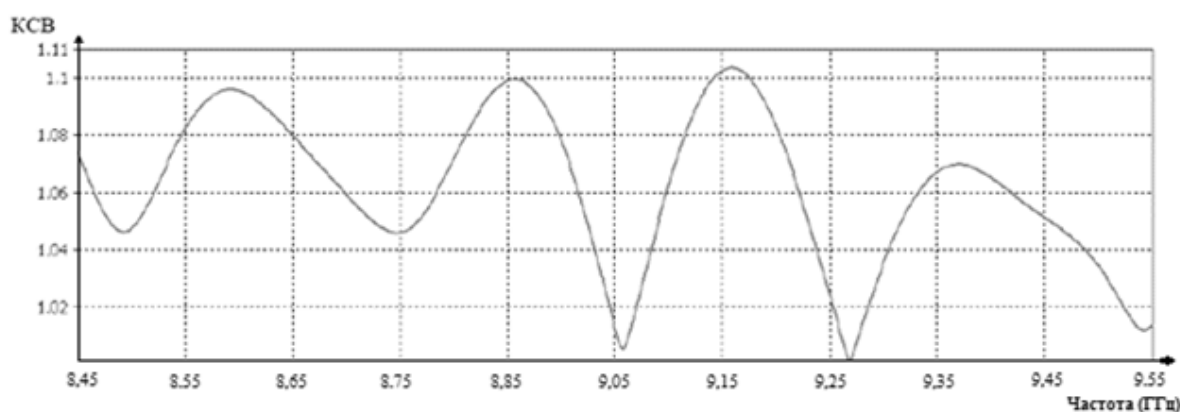
Рис. 1. График зависимости значений КСВ от частоты
