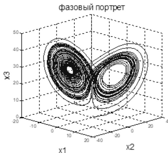
Рис. 1. Движение системы в фазовом пространстве
